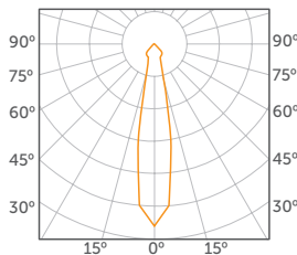
REFLECTOR CONCENTRADO 19°
