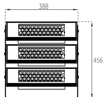
3 MÓDULOS 270W
