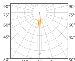
SUPER CONCENTRADA 10°
