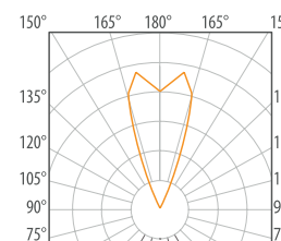
DIFUSA 40°
