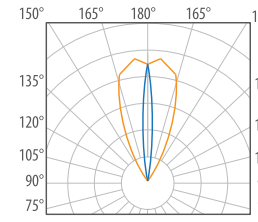
ELÍPTICA 17°x35°
