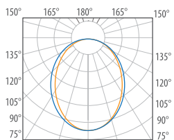
LUZ CONCÉNTRICA
