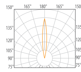
CONCENTRADA 14°
