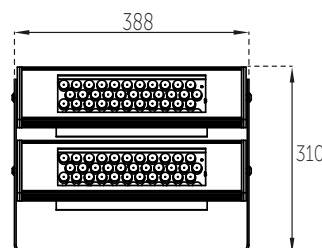
2 MÓDULOS 180W
