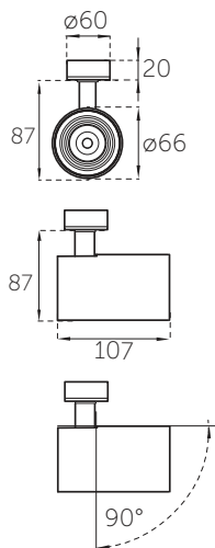
TRACK CÁNOPE
