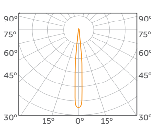
SUPER CONCENTRADA 10°
