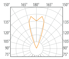
DIFUSA 40°
