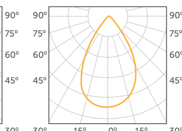
DIFUSA 60°
