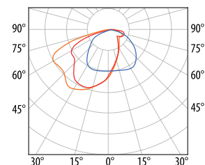
TIPO T4
