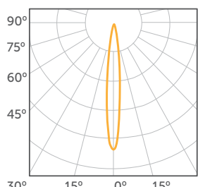
CONCENTRADA 11°
