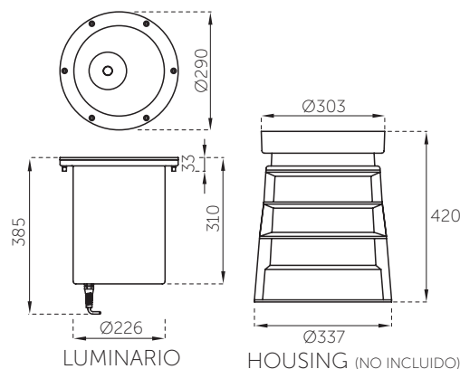
CUERPO DE ACERO INOXIDABLE
