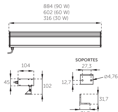
CONECTOR IP 68 (INCLUIDO)
