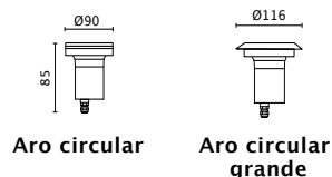
EMPOTRAR
